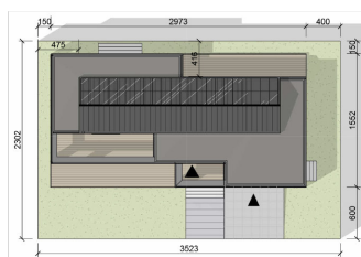
ZAGOSPODAROWANIE TERENU
